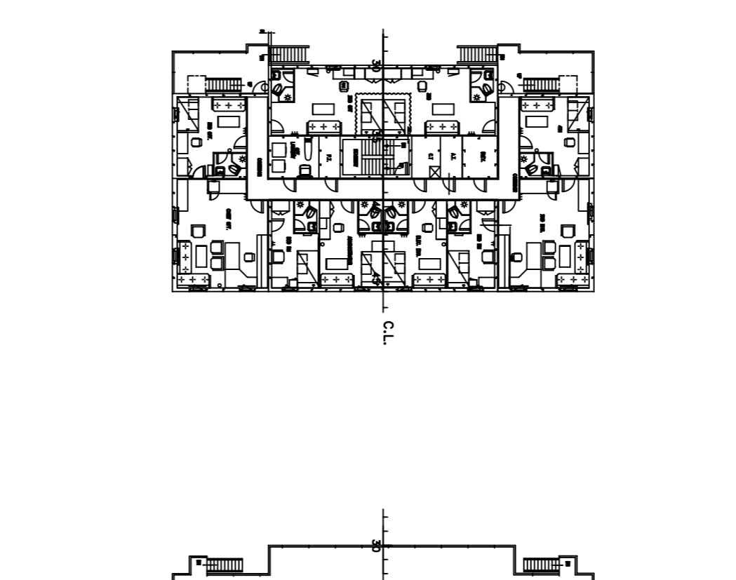
C-DECK
